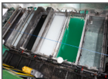
ディップ処理槽
