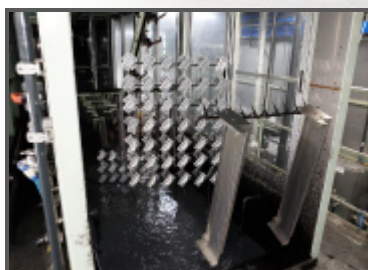
カチオン電着槽
